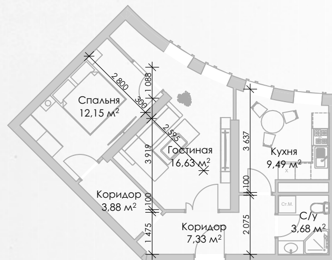
Двухкомнатная квартира 2А
