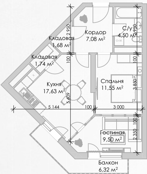
Двухкомнатная квартира 1Г
